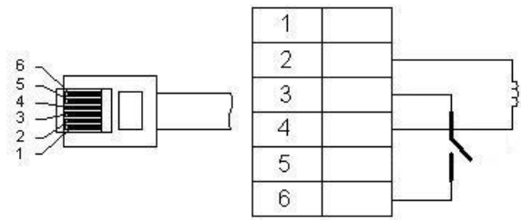
Электрическая схема управления денежным ящиком
