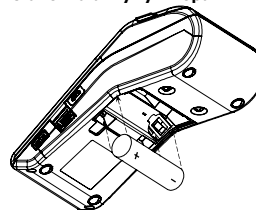
Рисунок 2. Установка аккумулятора
